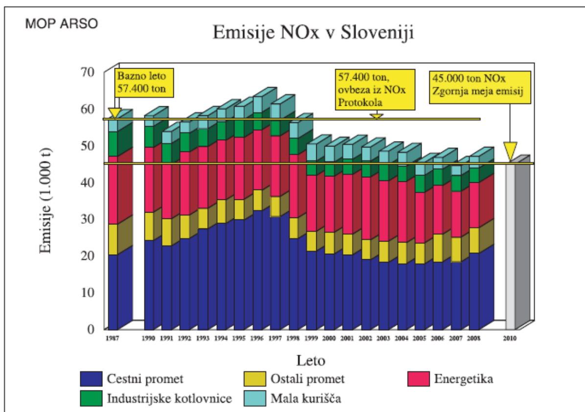
Slika 28: Izpusti dušikovitih oksidov NO x v Sloveniji
