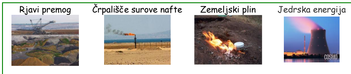
Slika 58: Neobnovljivi viri energije
