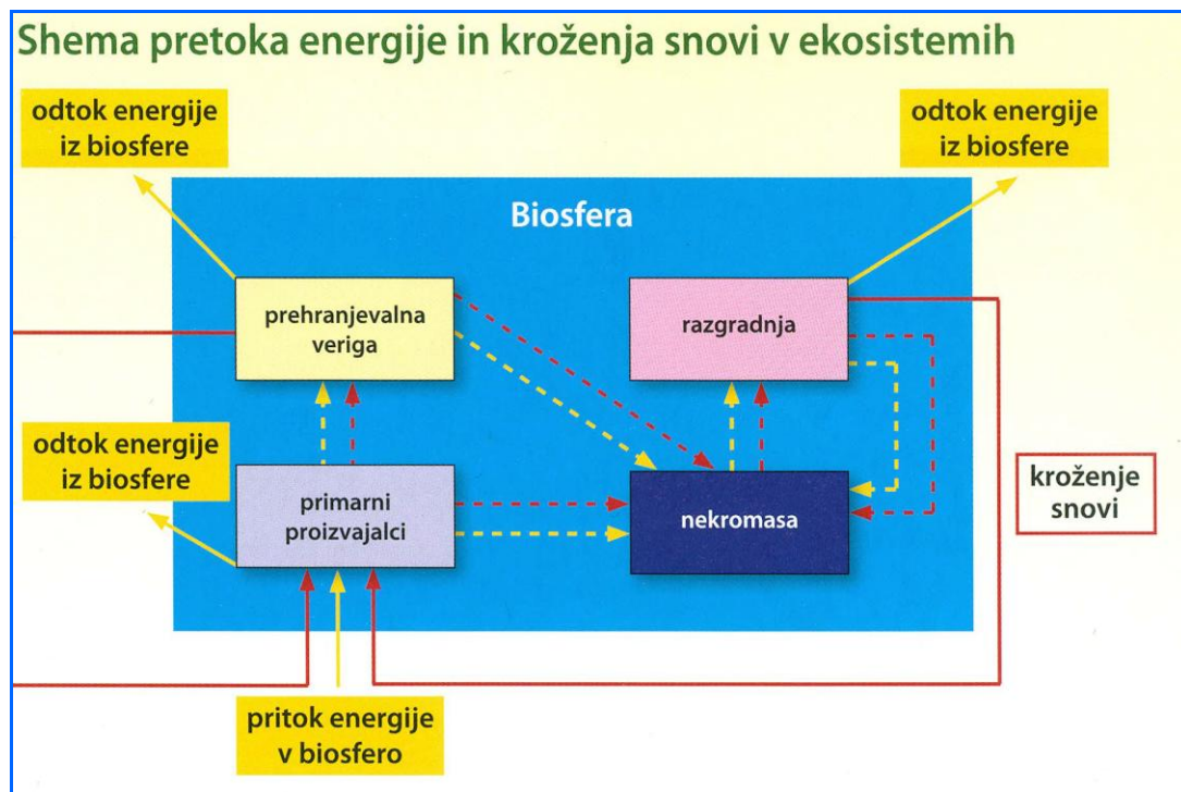
Slika 3: V ekosistemih sta snov in energija združeni skupaj v obliki energetske bogate organske snovi. Izven ekosistemov potujeta snov in energija ločeno.
