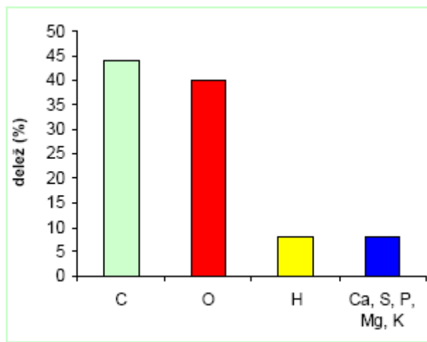
Slika 93: Elementarna sestava talne organske snovi
